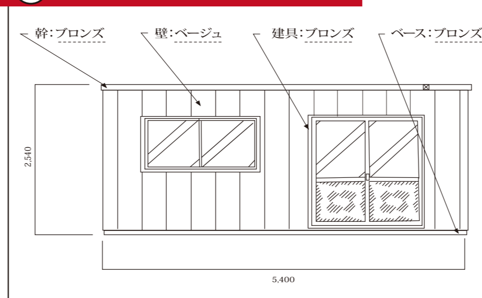
立面図 A SCAL=1:40 M
