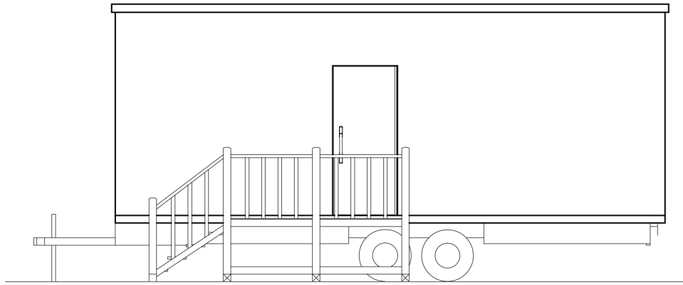
立面図 ①
